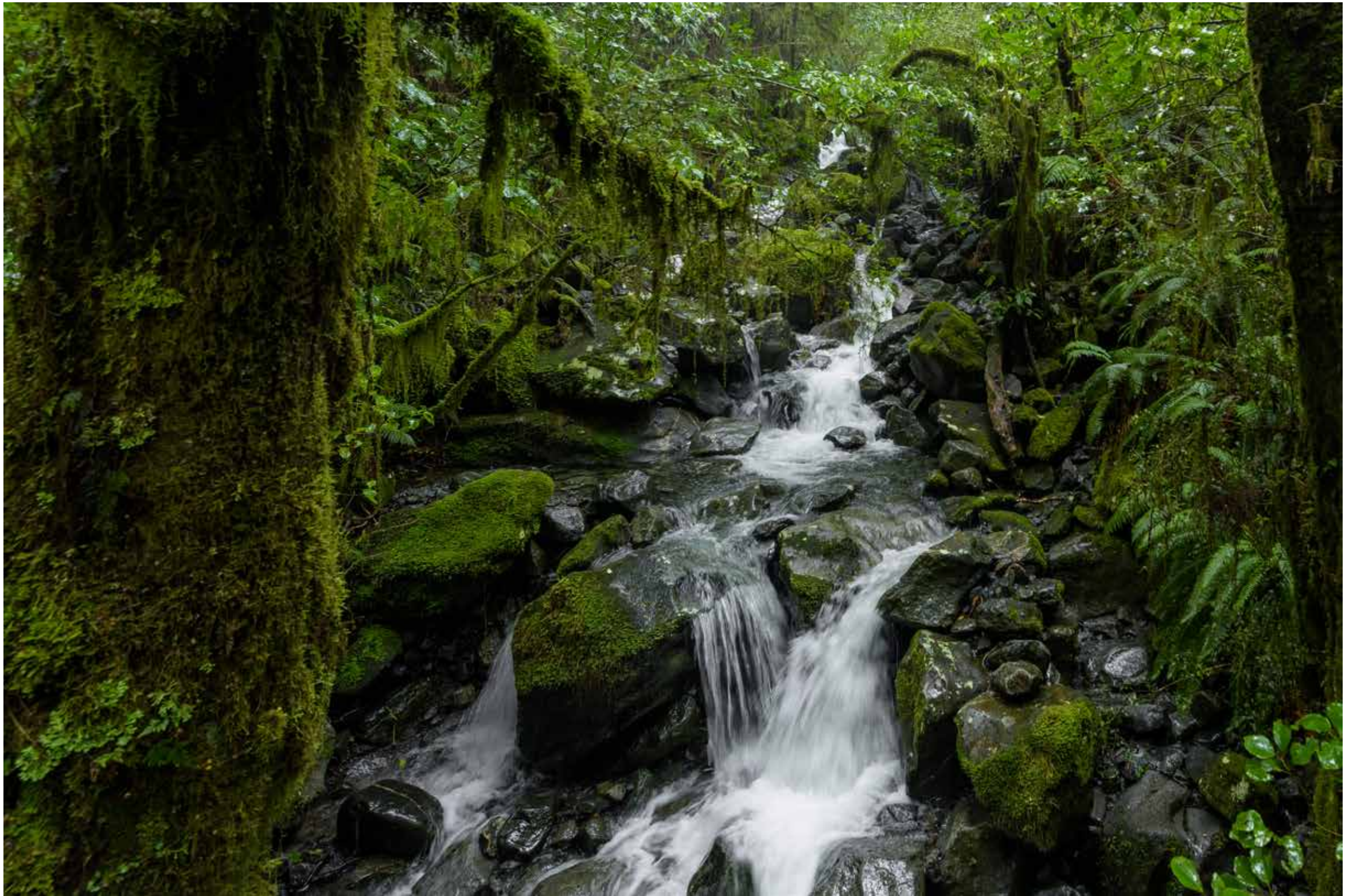
"Selva neozelandesa" - Southland, Nueva Zelanda
